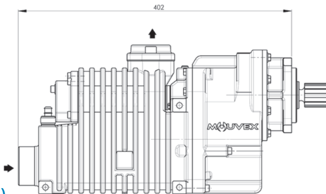
Version: Am Nebenantrieb direkt angeflanscht (PF)
