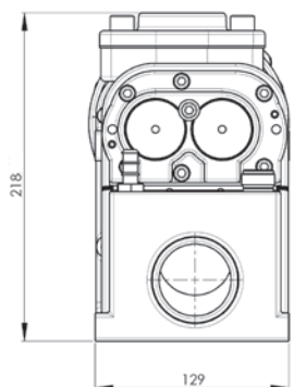
Version: Am Nebenantrieb direkt angeflanscht (PF)
